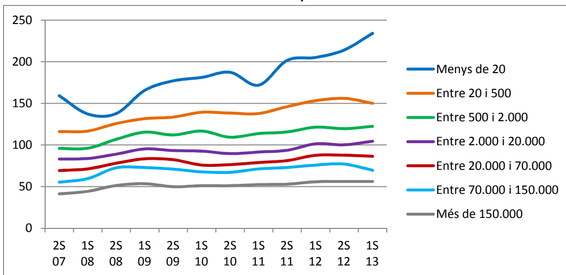
Preu sense IVA de l'electricitat en funció del consum en MWh per any a Espanya (€ per MWh)
